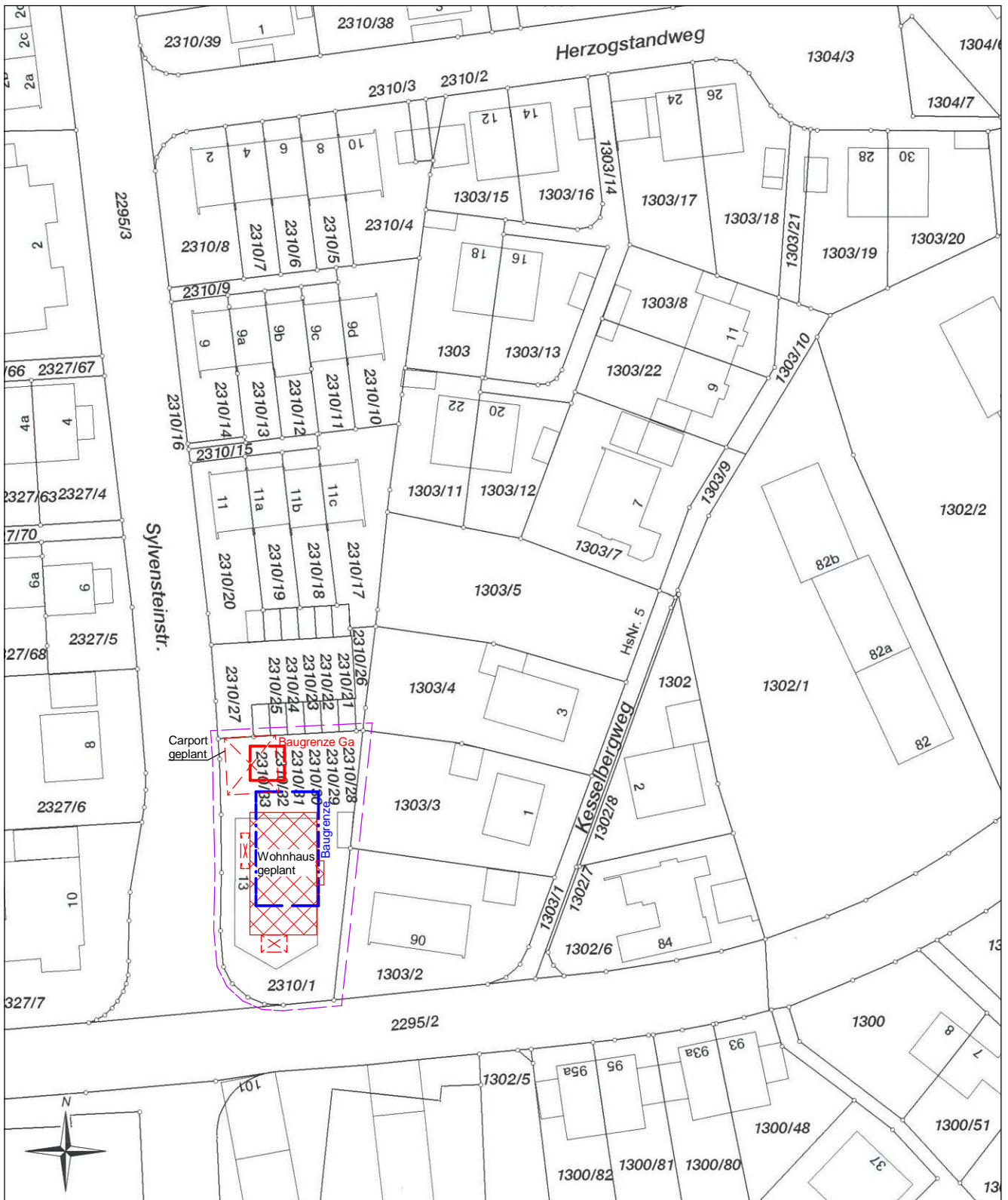
Lageplan M 1:1000
