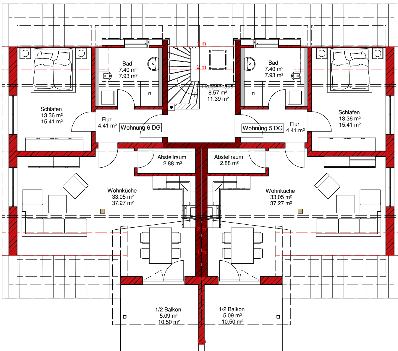
Dachgeschoss
