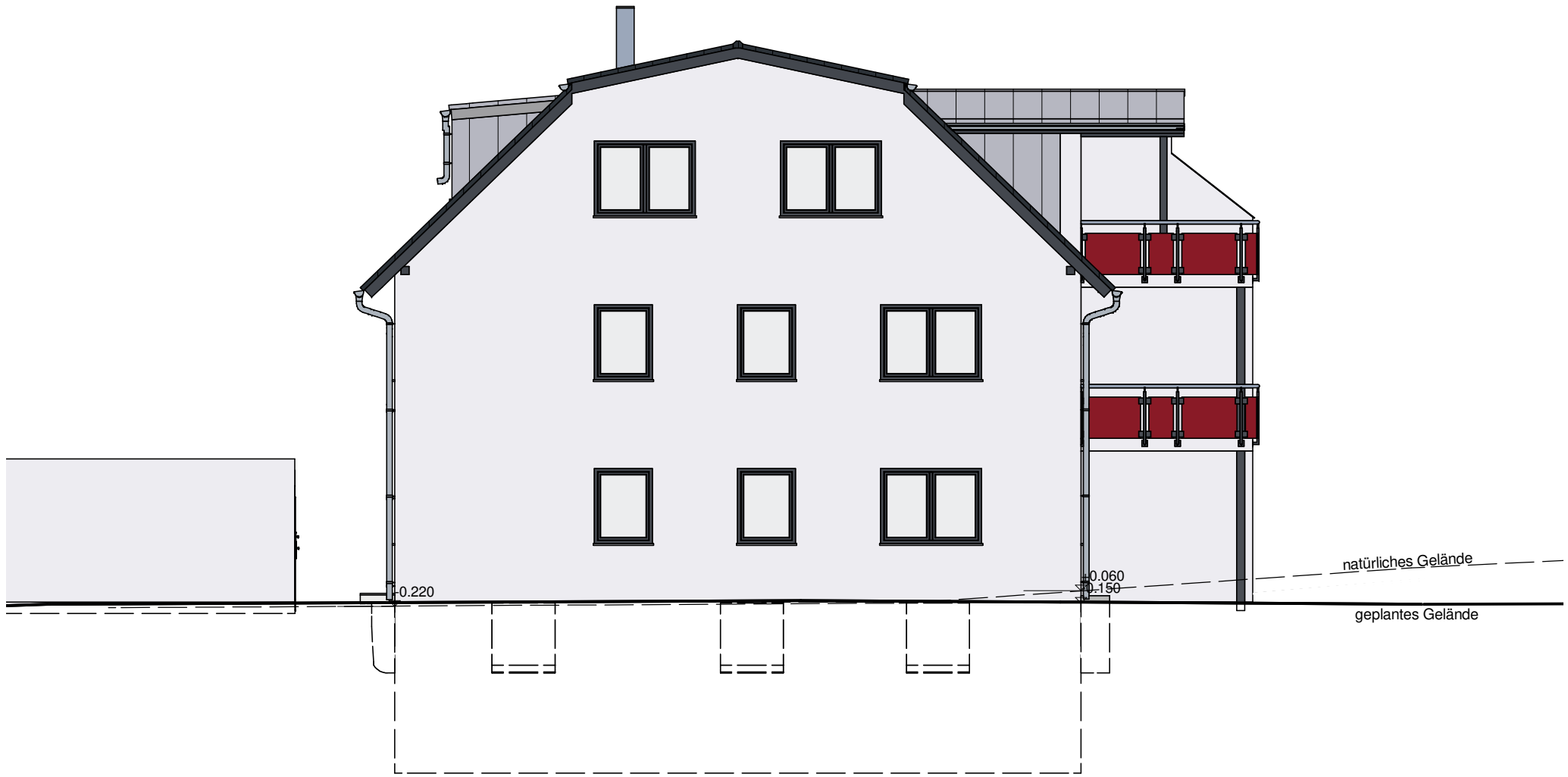
Ansicht West
