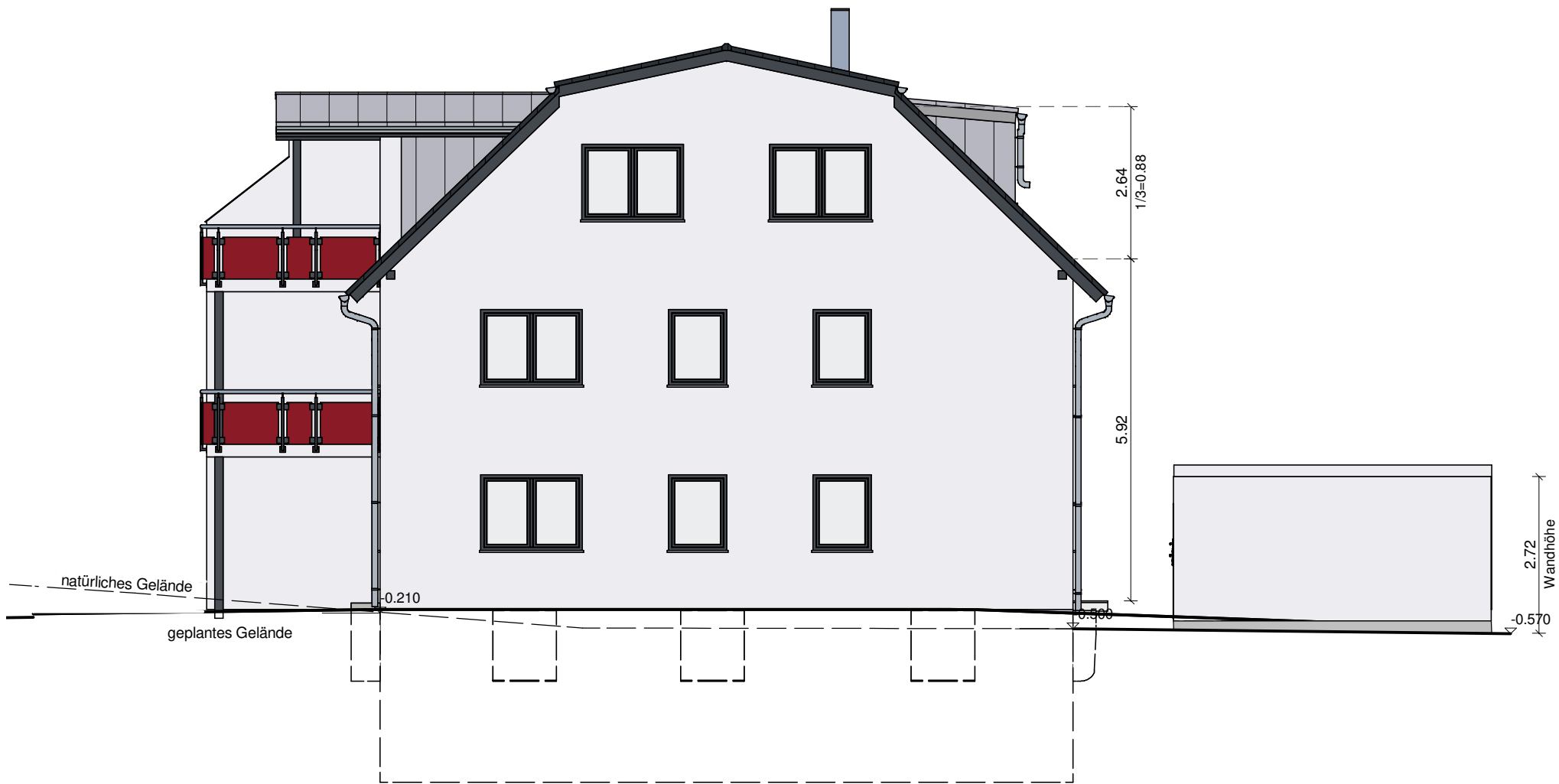
Ansicht Ost
